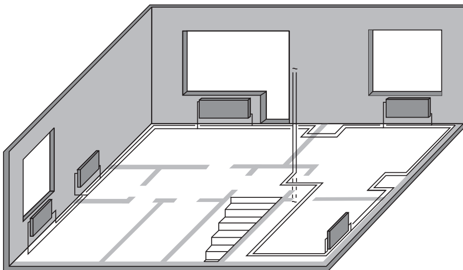
Рис. 13. Двухтрубная система с горизонтальными компенсирующими петлями
