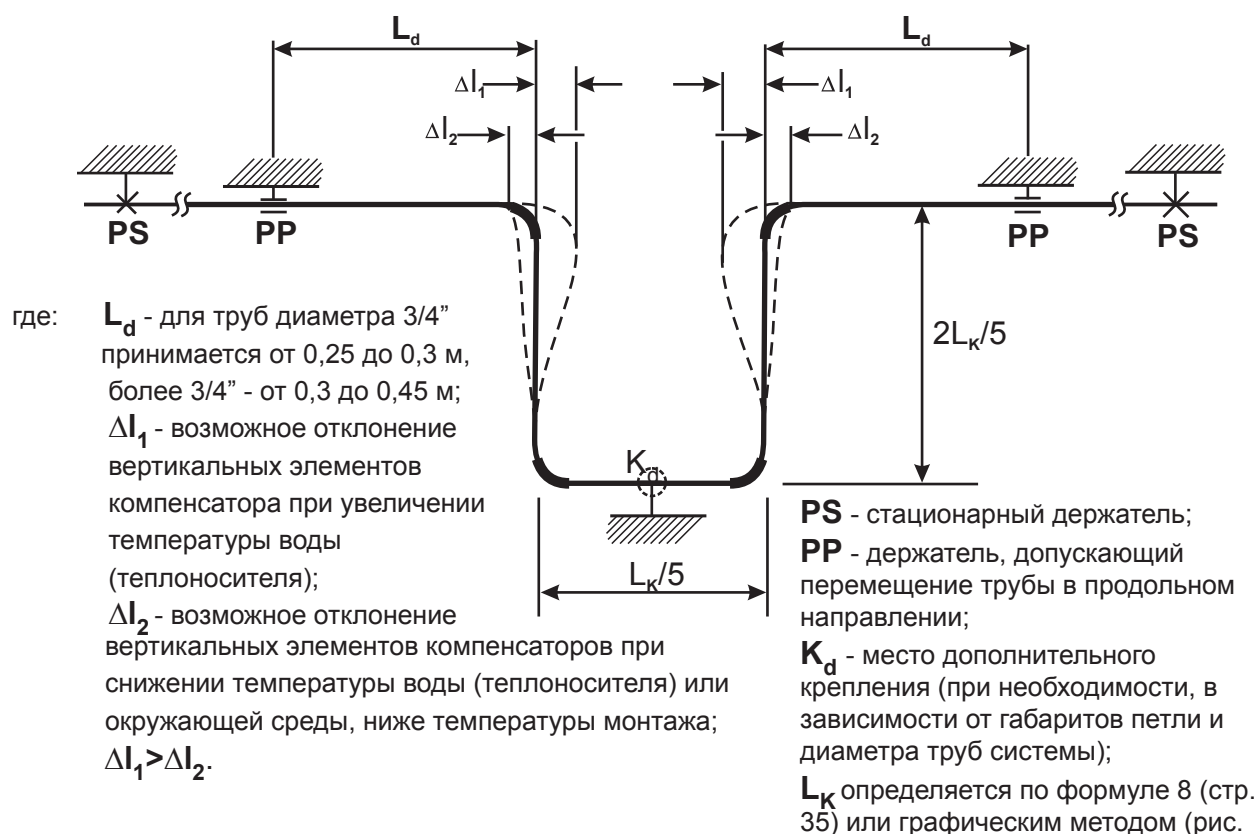
Рис. 38. Компенсирующая петля («U» образный компенсатор) и места установки держателей
