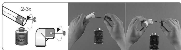
Рис. 27. Нанесение клея на склеиваемые элементы
