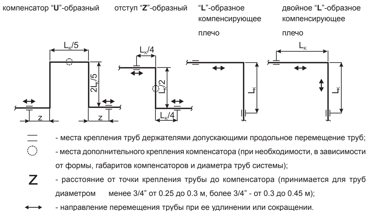
Рис. 9. Рекомендуемые конструкции компенсаторов
