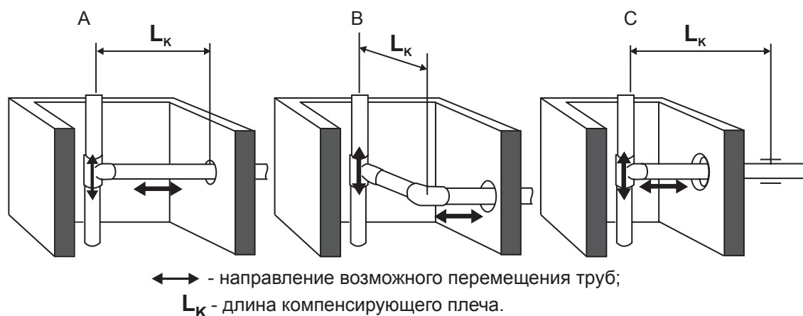
Рис. 40. Возможные конструкции компенсаторов в нормальных (А, В) и узких (С) каналах
