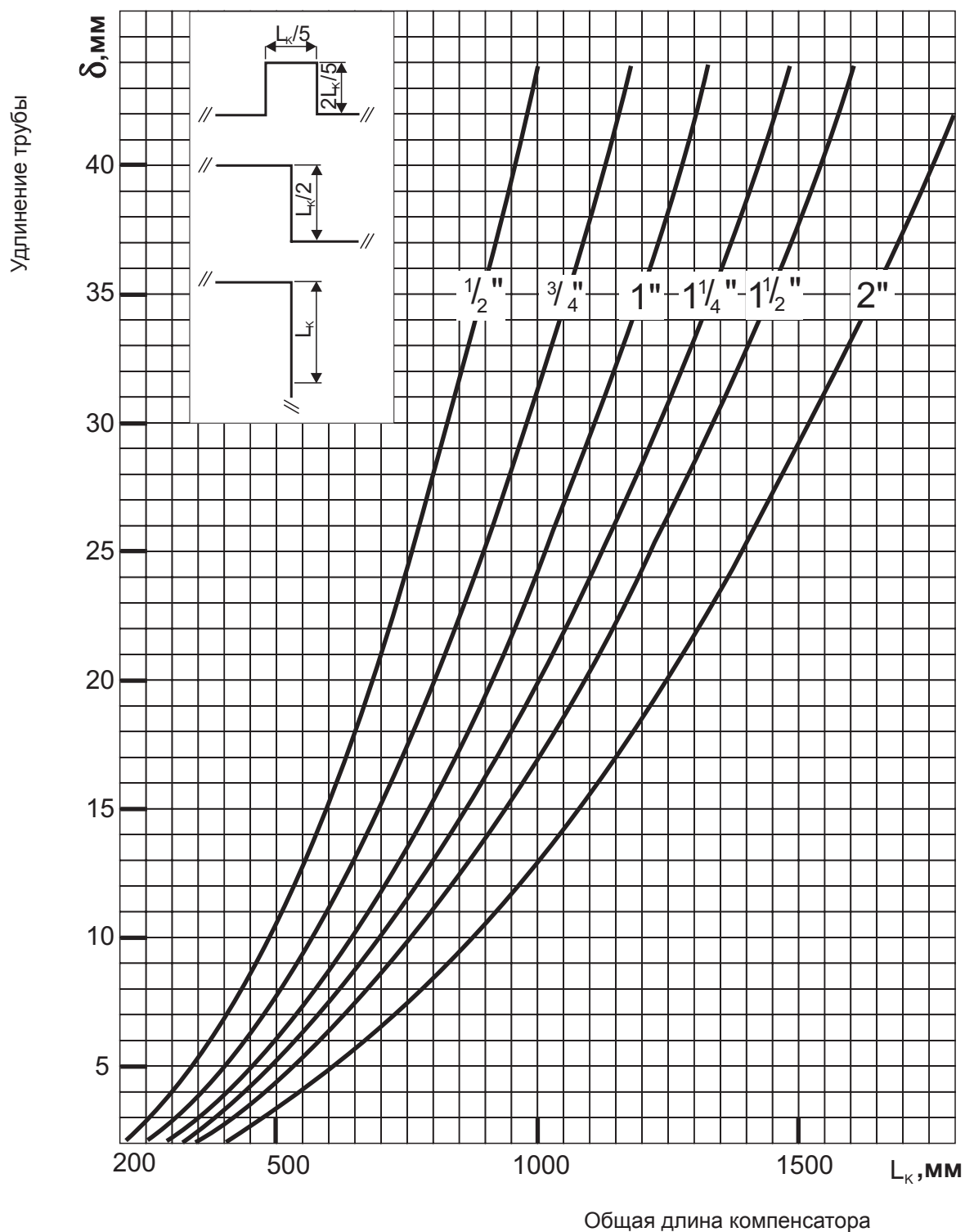
Рис. 10. Размеры компенсаторов для систем водяного отопления ( t_p = 80^\circ\text{C} ; t_m = 10^\circ\text{C} ), где: t_p - рабочая температура теплоносителя; t_m - температура окружающей среды во время монтажа системы.
